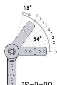
IS-9-90 zero position= 90° end position= 144°
