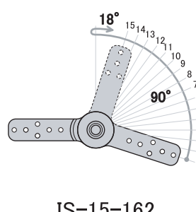
IS-15-162 zero position=162° end position= 252°
