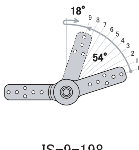
IS-9-198 zero position=198° end position= 252°
