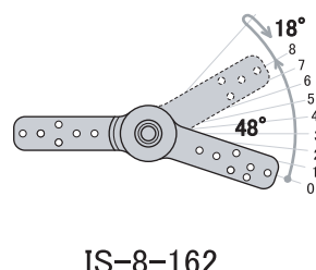
IS-8-162 zero position=162° end position= 210°
